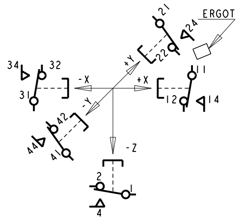
SCHEMA ELECTRIQUE VUE DE DESSUS
